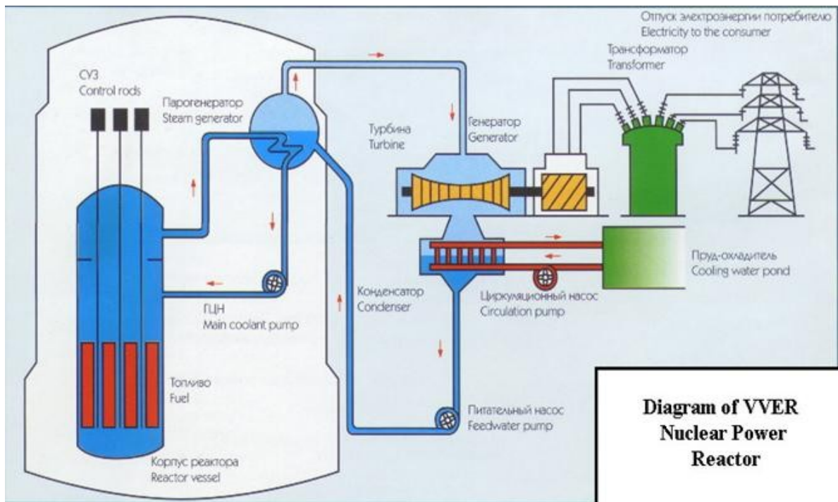
Ábra: Paks bővítésére, a Rusatom által tervezett VVER rektor működése.
