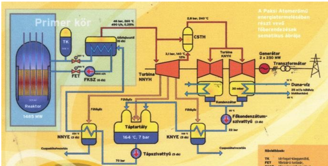
8.Ábra: A 4 előregedett reaktor jelenlegi működése
